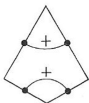
IH31 [3 . 4 . 6 . 4]
