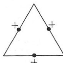
IH84 [6^3]
