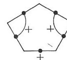
IH28 [3^2 . 4 . 3 . 4]
