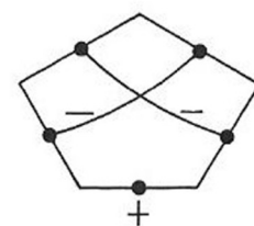
IH27 [3^2 . 4 . 3 . 4]
