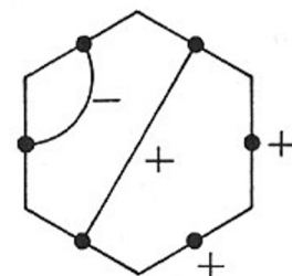
IH5 [3^6]
