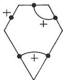
IH21 [3^4 . 6]
