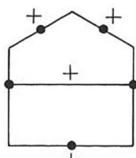
IH23 [3^3 . 4^2]
