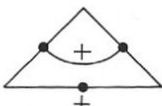
IH79 [4 . 8^2]
