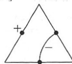
IH28 [3^2 . 4 . 3 . 4]
